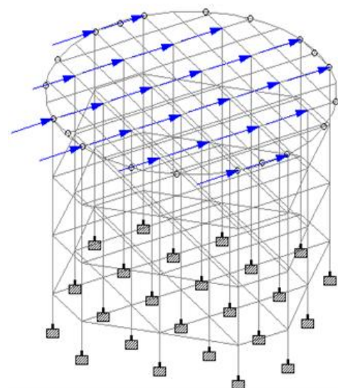
Fig. 4- Seismic Load
