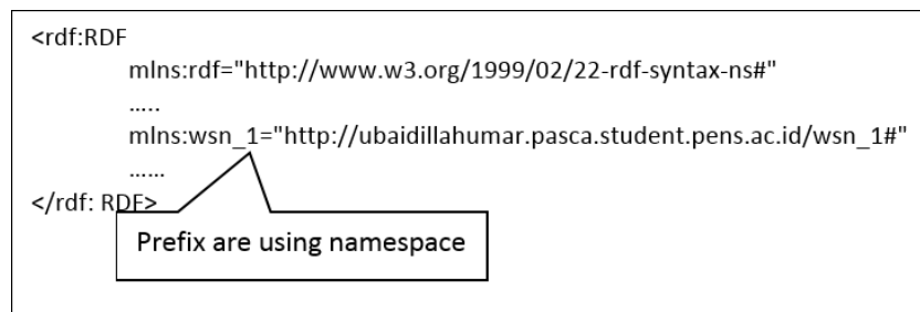
Fig. 9 Namespaces prefix
