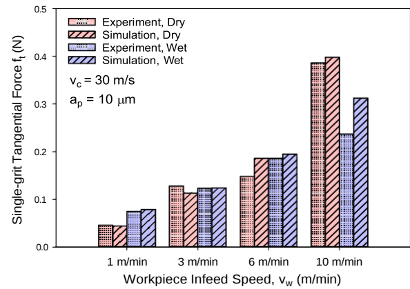
(d) Single-grit tangential force vs. workpiece infeed speed
