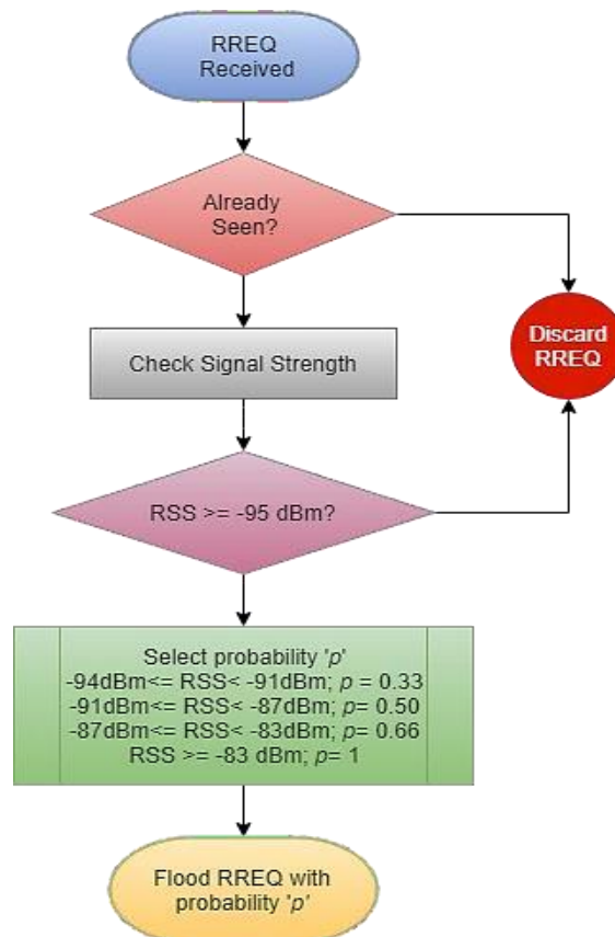
Fig. 1 CQAG-AODV flowchart
